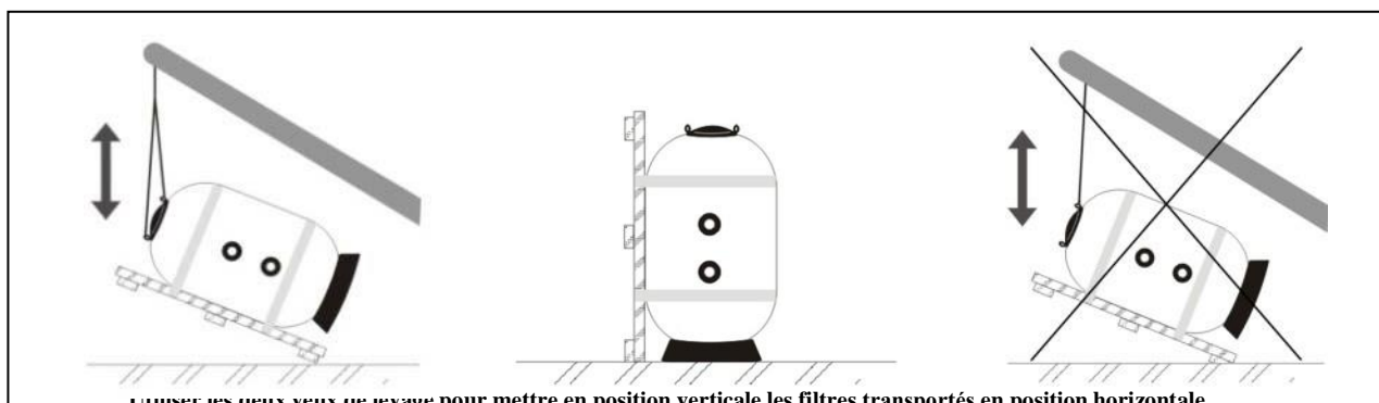
Insérer les yeux yeux de levage pour mettre en position verticale les filtres transportés en position horizontale
