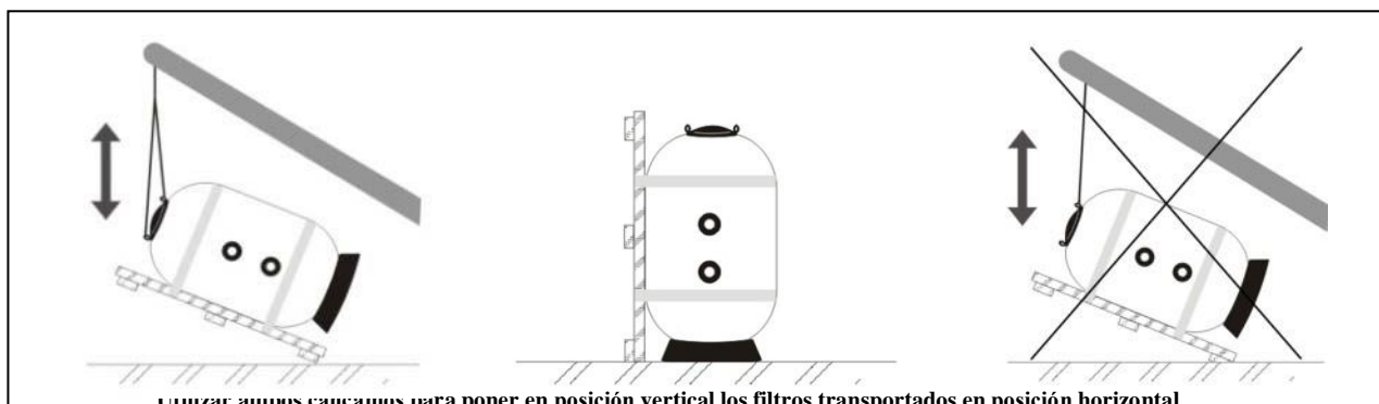
Utilizar ambos caucho para poner en posición vertical los filtros transportados en posición horizontal
